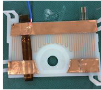
図 5. 熱電対と銅テープの貼り付け状態
