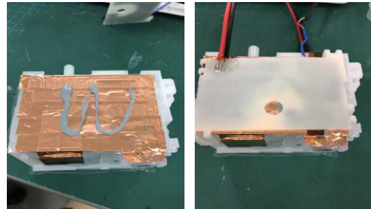
図 6. 熱伝導グリスを塗ったヒーター部
