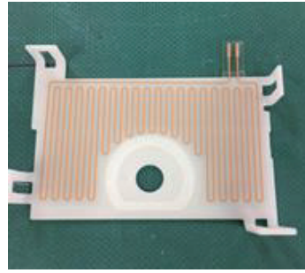
図 4. ヒーターの貼り付け状態
